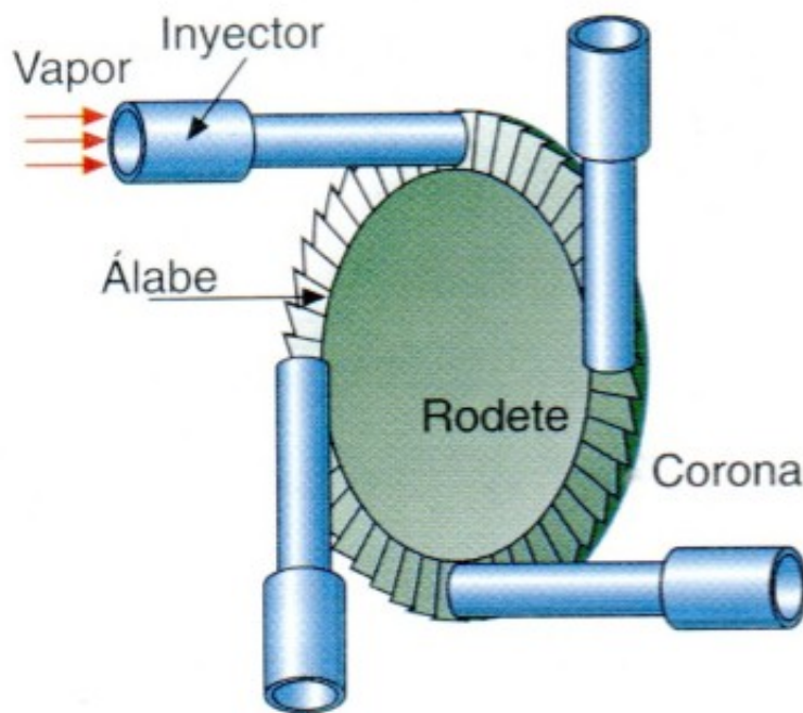
Turbina de vapor.
